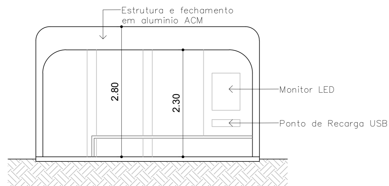
ELEVAÇÃO FRONTAL escala 1:50
