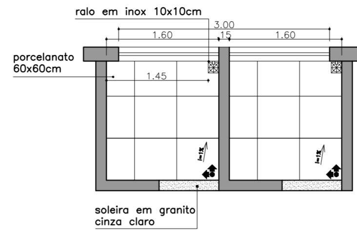
PLANTA PAGINAÇÃO PISO esc 1:50
