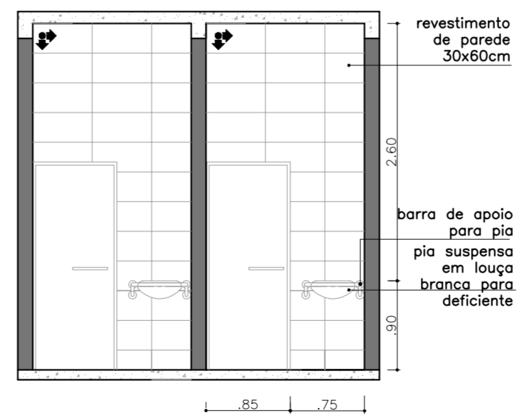
VISTA 4 esc 1:50
