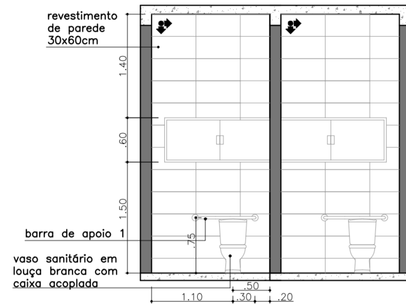
VISTA 1 esc 1:50
