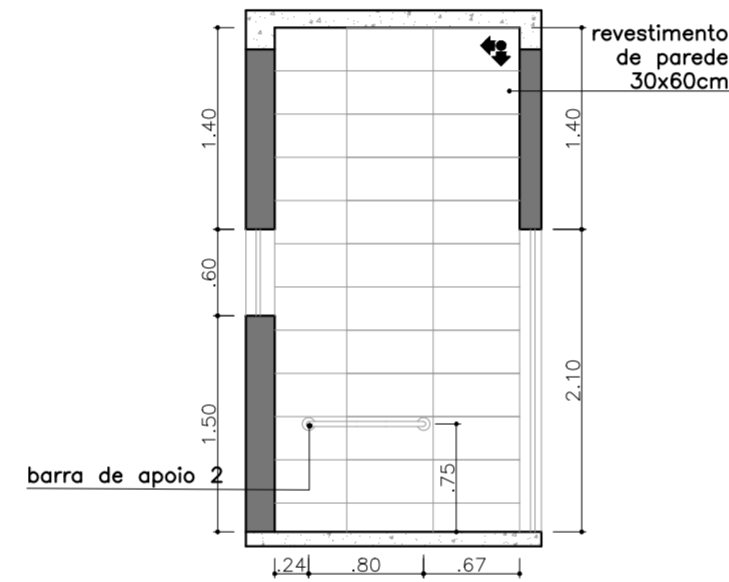
VISTA 2 esc 1:50
