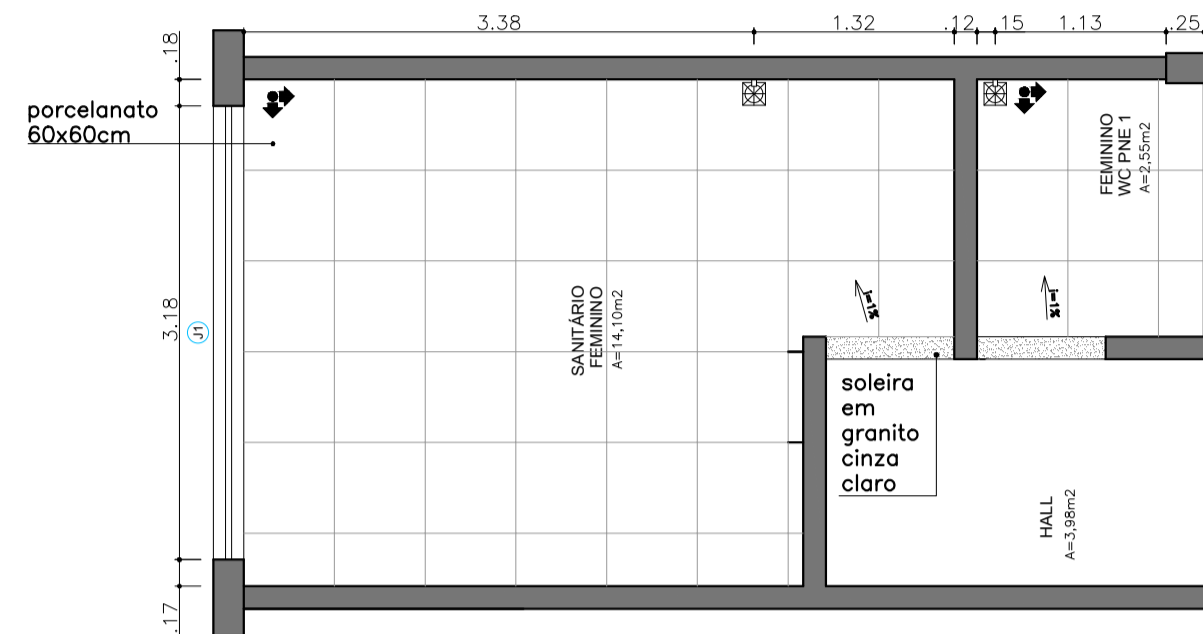
PLANTA PAGINAÇÃO PISO esc 1:50
