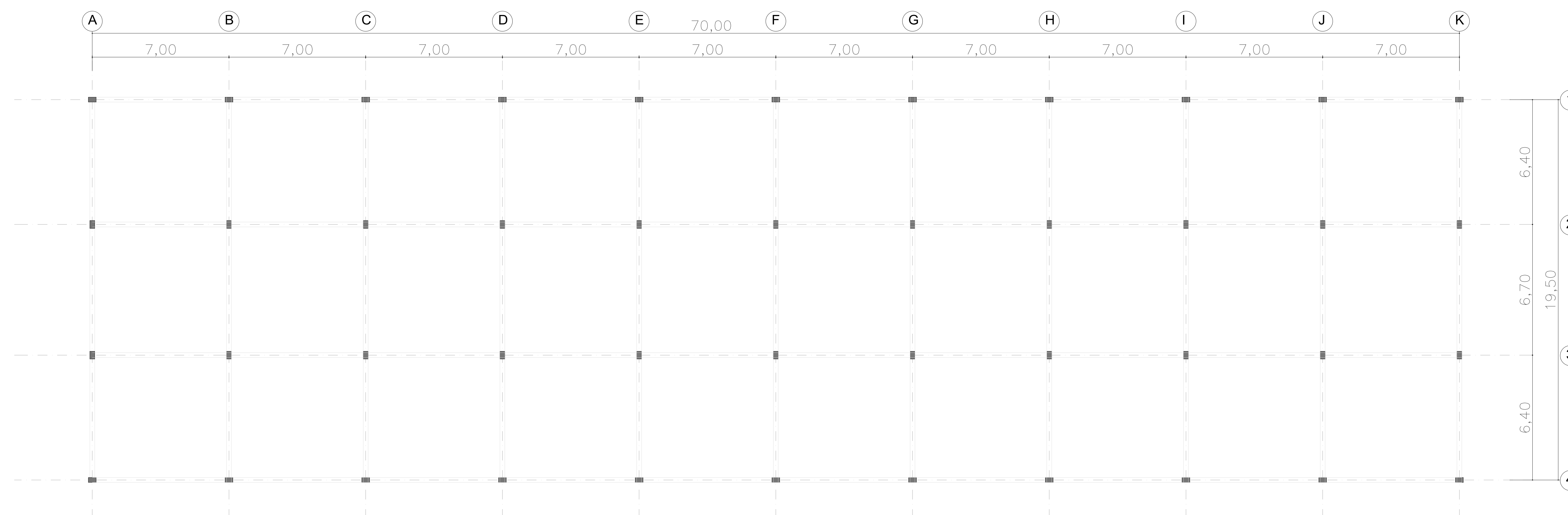
PLANTA NÍVEL COBERTURA VIGAS 0,15X0,40 ESCALA 1:100
