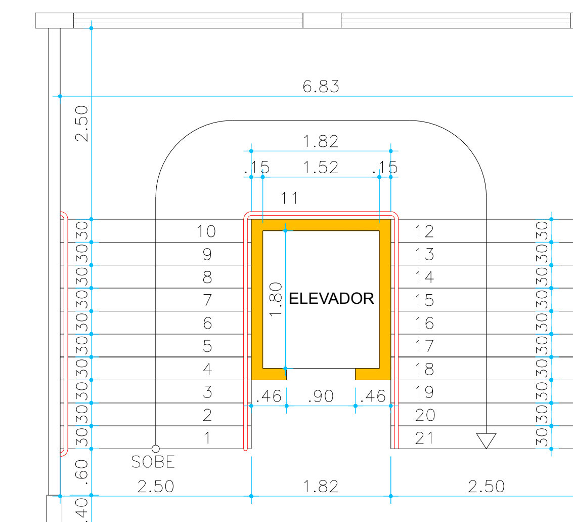
DET. ESCADA ESCALA 1:100
